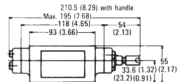
( ) dimensions for the OCY-G03-X-J50.
