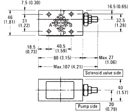
( ) dimensions for the OCY-G01-B-X-(E)20.
