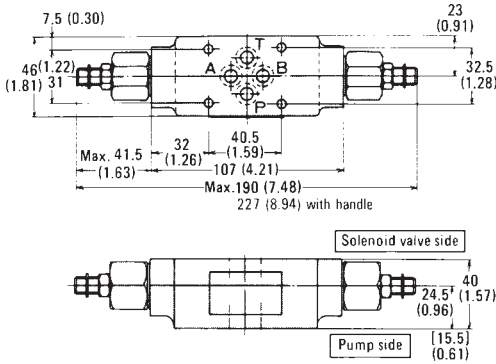
( ) dimensions for the OCY-G01-W-X-(E)20.
