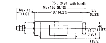
( ) dimensions for the OCY-G01-A-X-(E)20.
